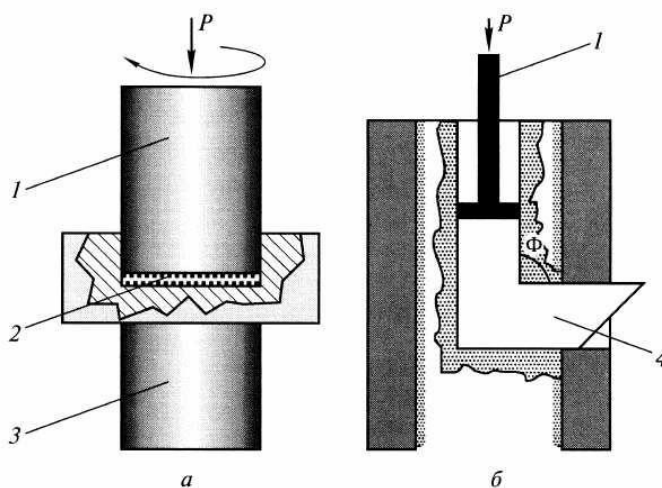
Рисунок 3.1 - Схема методів інтенсивної пластичної деформації: а- метод крутіння під високим тиском, б- метод рівноканального кутового пресування.
